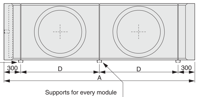
HTC-N 076 / 090 / 091 / 100 . 1•• Horizontal Air Direction
